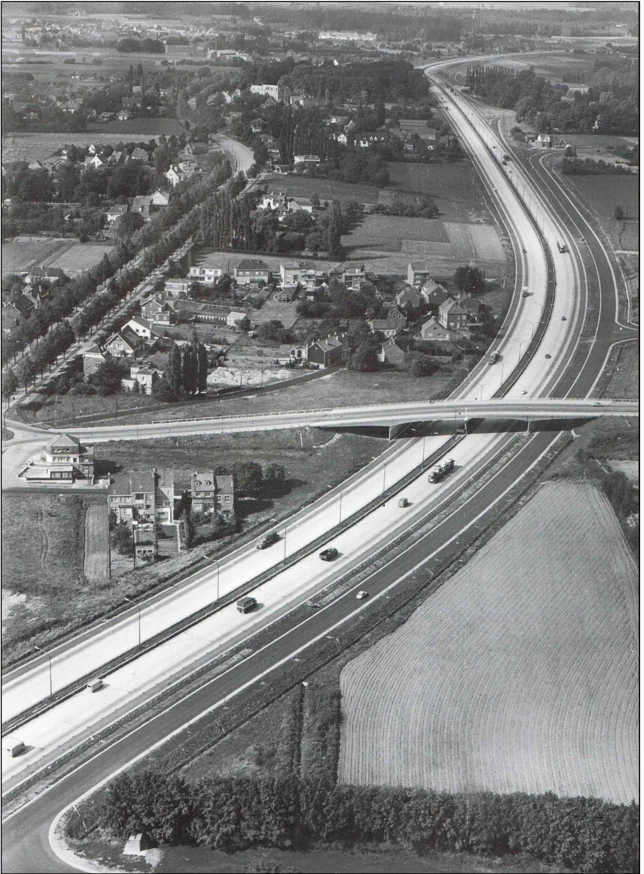
Luchtfoto met een nieuw-aangelegde A-12 en de nog nieuwe brug van de Kapellelaan.
